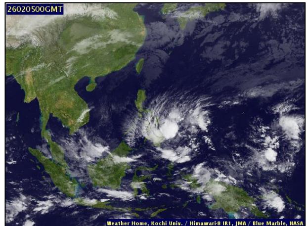
ภาพถ่ายดาวเทียม วันที่ ๕ ก.พ. ๒๕๖๙ เวลา ๐๗.๐๐ น.
